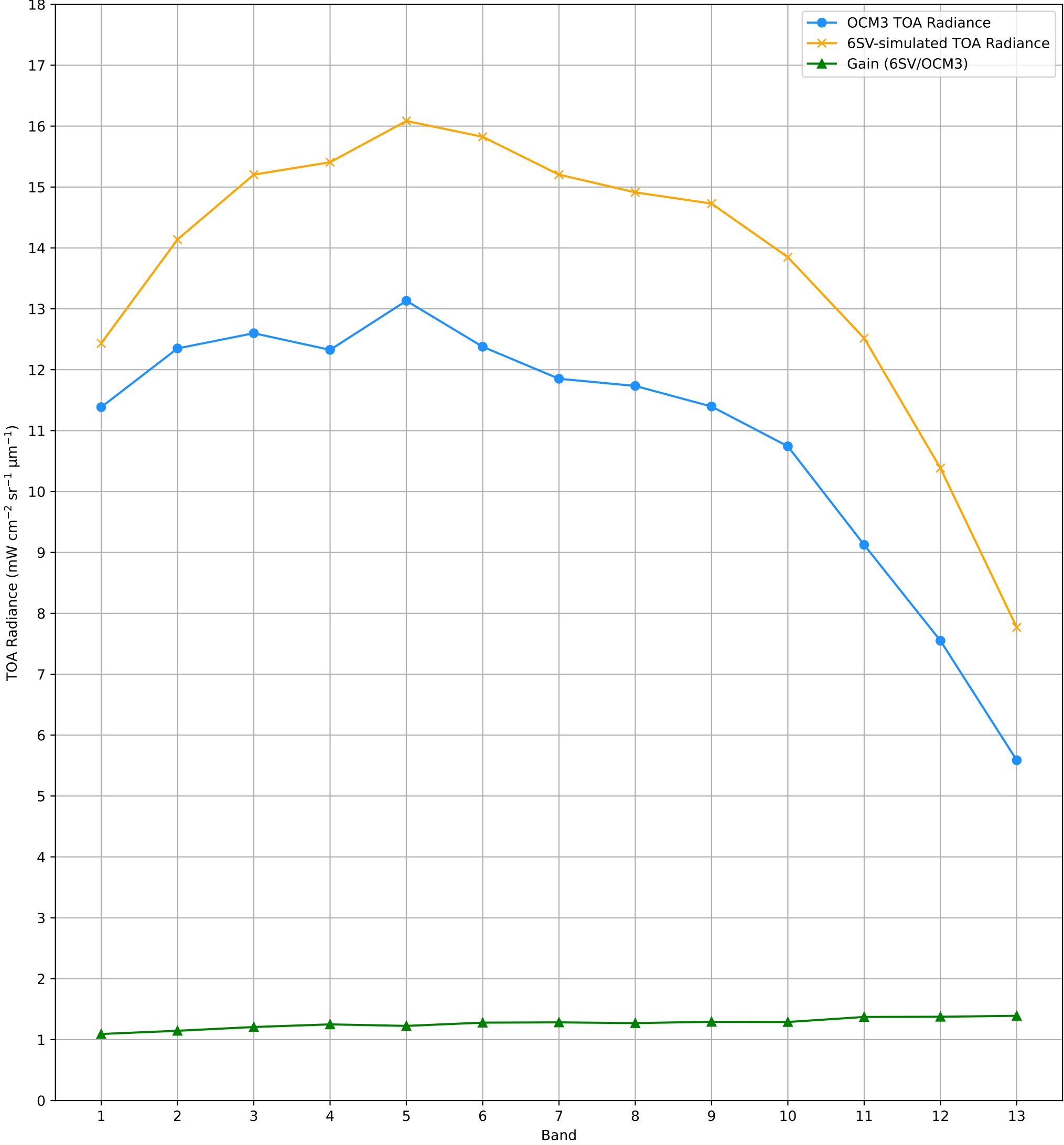
TOA Radiance (OCM3 vs. 6SV) over RVUS RadCalNet Site Lat: 38.497°, Lon: -115.69° - 29-AUG-2025 (STRIP_ID: 14572)
