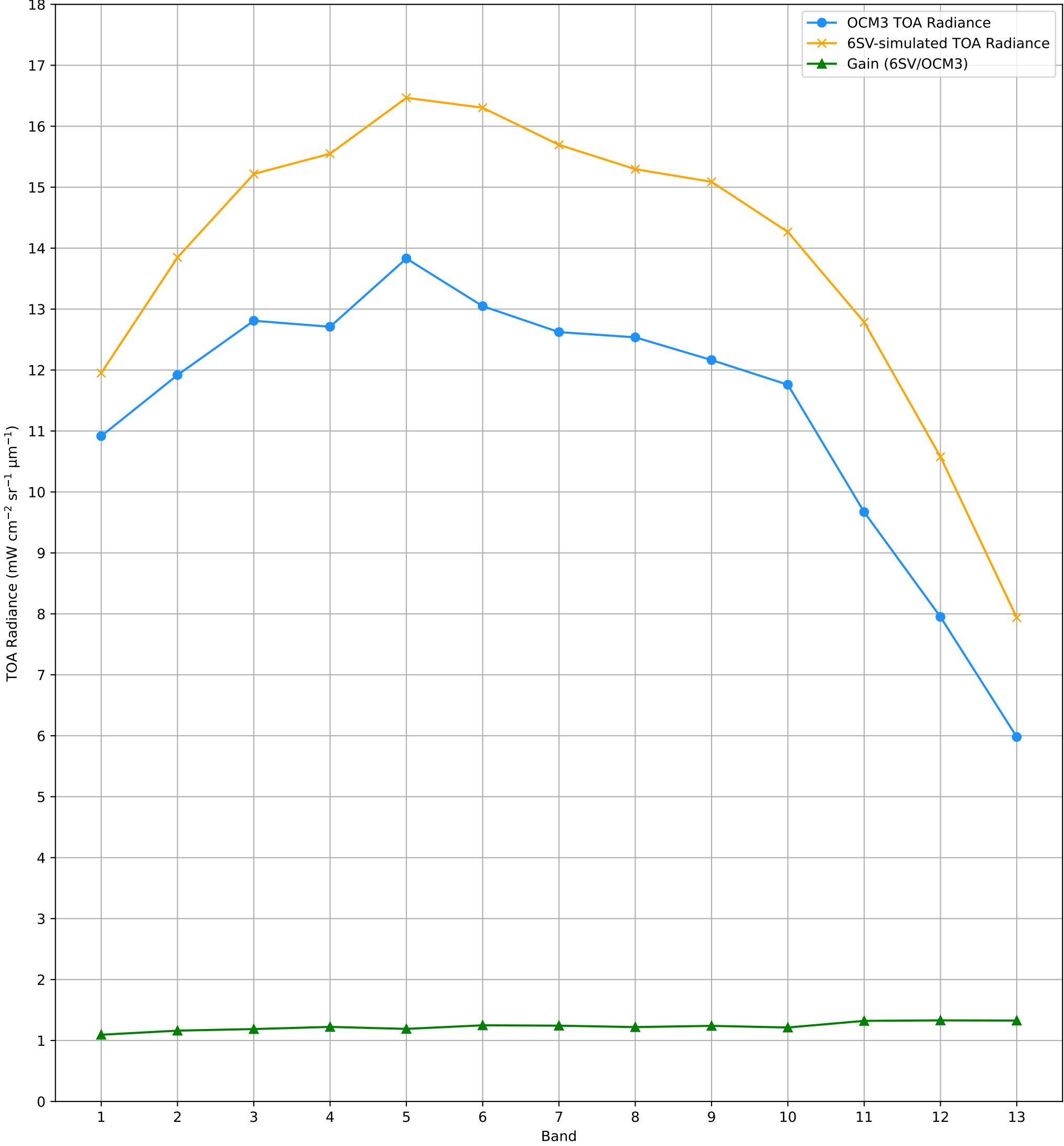
TOA Radiance (OCM3 vs. 6SV) over RVUS RadCalNet Site Lat: 38.497°, Lon: -115.69° - 30-AUG-2025 (STRIP_ID: 14586)
