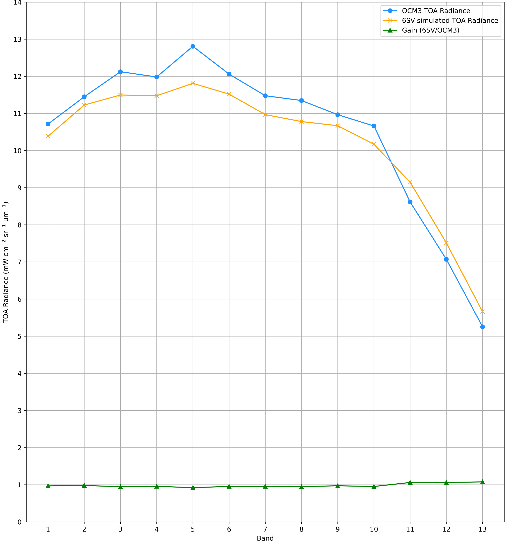
TOA Radiance (OCM3 vs. 6SV) over RVUS RadCalNet Site Lat: 38.497°, Lon: -115.69° - 01-NOV-2025 (STRIP_ID: 15497)
