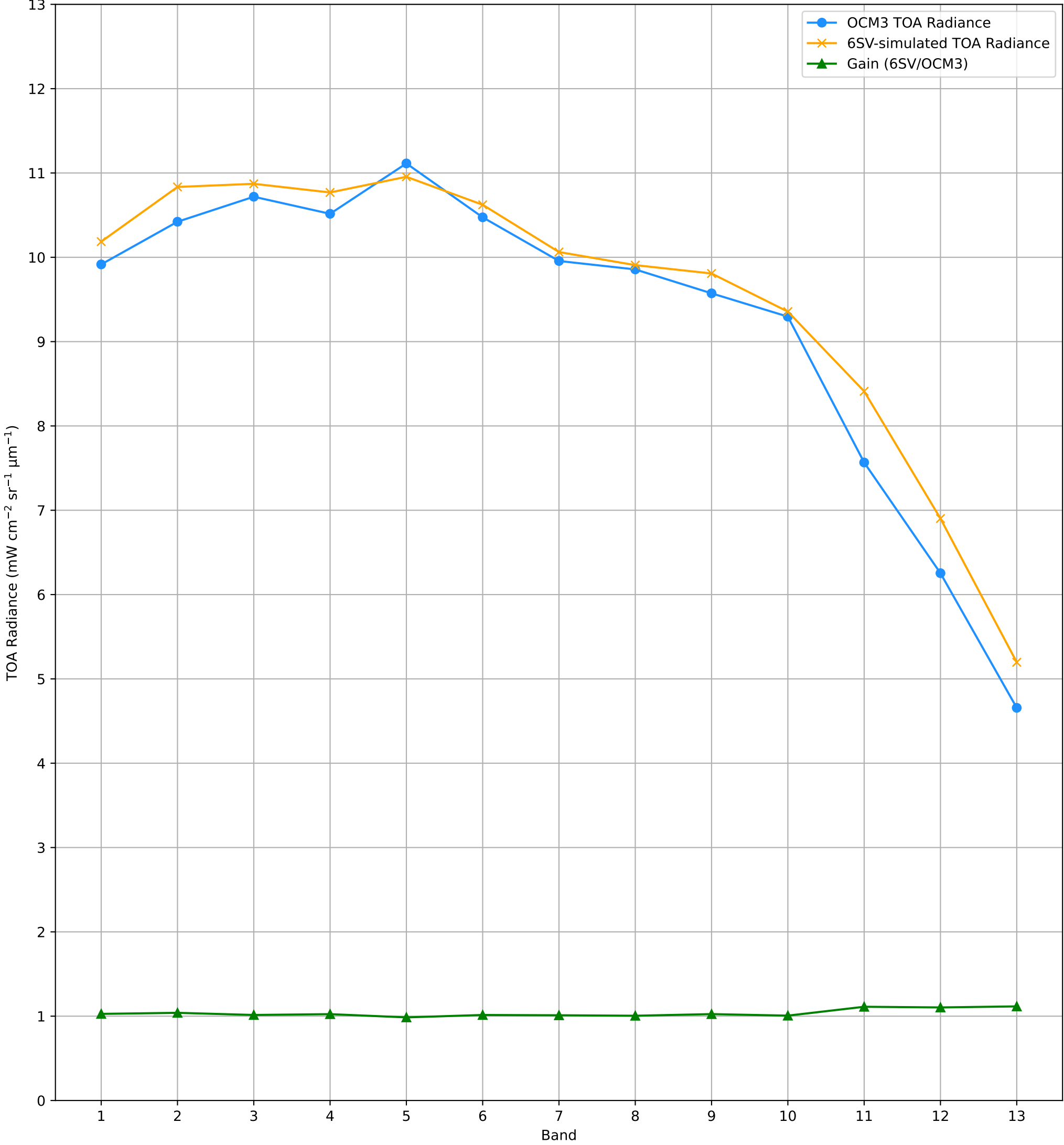
TOA Radiance (OCM3 vs. 6SV) over RVUS RadCalNet Site Lat: 38.497°, Lon: -115.69° - 02-NOV-2025 (STRIP_ID: 15512)
